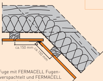
Bild 9: 1. Spachtelfuge mit aufgeklebtem FERMACELL Gewebeband oder einem eingespachtelten Papiereckband
