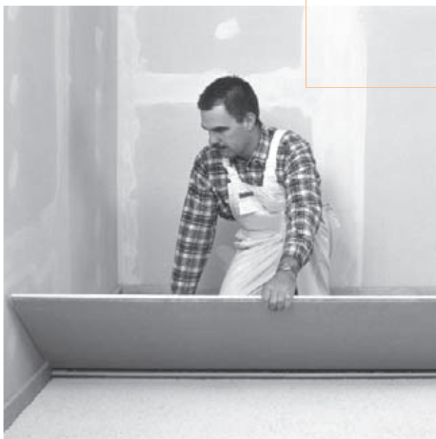
Bild 44: Das trittschall- und wärmedämmende FERMACELL Estrich-Element. Im Format 150 x 50 cm. In neun verschiedenen Dicken und Ausführungen lieferbar.
