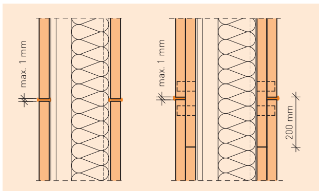
Horizontale Klebefuge
