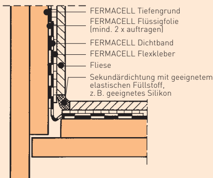
Bild 36: Wand-Eckausbildung im wasserbeanspruchten Bereich
