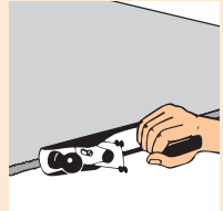
Bild 5: Glatthobeln der Bruchkante von Plattenzuscchnitten bei Sichtkanten
