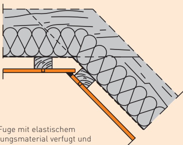
Bild 11: 3. Elastische Fuge (z. B. Acryl)
