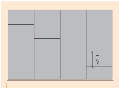
Bild 24: Verlegung im schleppenden Verband
