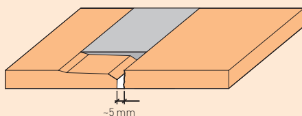
Bild 28: Fugenvariante 3: Eine werkseitige TB-Kante und eine bauseits zugeschnittene Kante und FERMACELL Fugenspachtel
