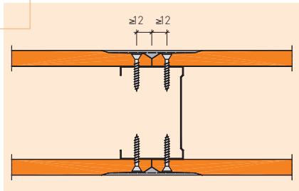
Bild 25: Nicht tragende Montagewände
