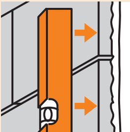
Bild 18: Die Platte wird leicht an die Wand gedrückt und durch Anklöpfen mit dem Richtscheit planeben ausgerichtet
