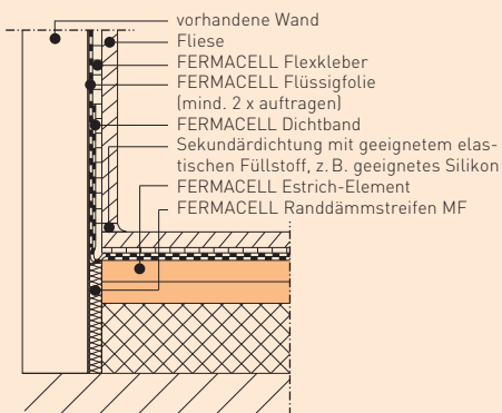
Bild 35: Wand-Estrichausbildung im wasserbeanspruchten Bereich
