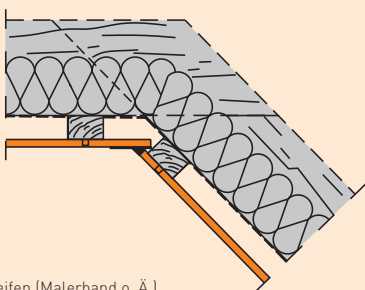
Bild 10: 2. Spachtelfuge mit Trennstreifen
