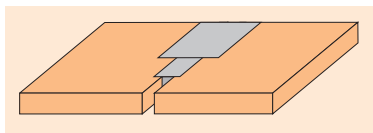
Bild 19: Fugenbreite in Abhängigkeit von der Plattendicke
