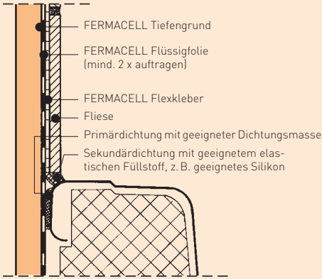
Bild 37: Wandanschlüsse von Dusch- bzw. Bader- wannen, Anschluss an FERMACELL Montage- wand einlagig beplant
