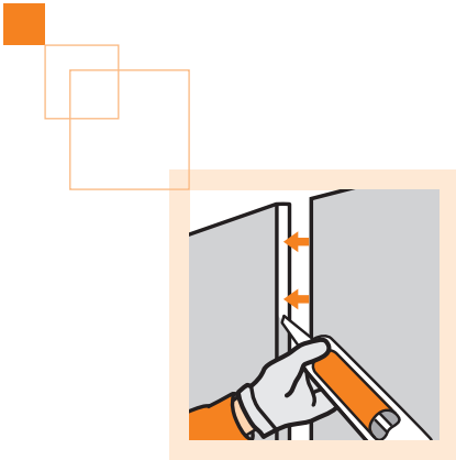
Bild 23: Führen der 310-mm-Kartusche an der Plattenkante. Die spezielle Kleberspitze sorgt für die exakte Klebermenge bei 10- und 12,5-mm-Platten. Bei 15- und 18-mm-Platten muss die Spitze angeschnitten werden.
