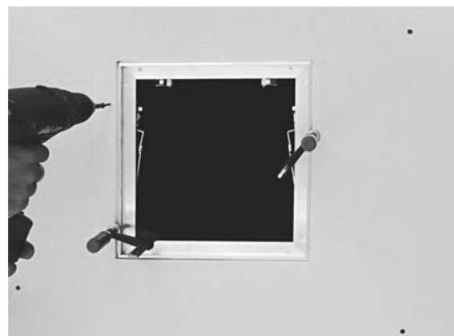
4. Rahmen verschrauben und beiliegende Schutzkappen aufstecken
