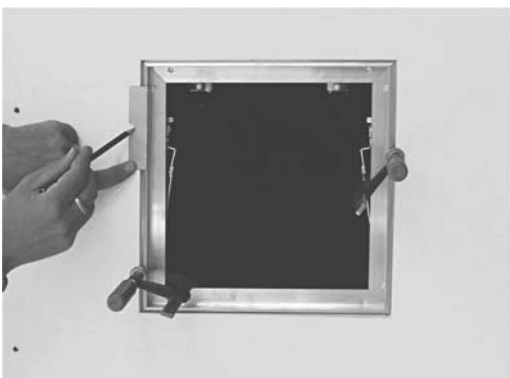
3. Rahmen ausrichten (Winkligkeit prüfen), festspannen und Bohrungen mit Schablone anzeichnen, Bohrabstand <100 mm
